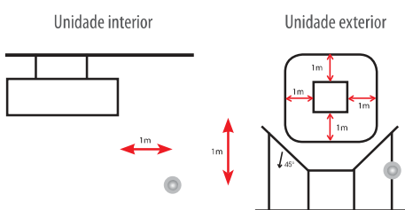
Medição pressão sonora- Standard JIS B8616-2006
